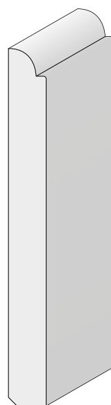
Londra sez. 18x170 mm
