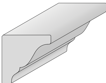
MOB 01: sez. 25x28 mm MOB 02: sez. 34x34 mm MOB 03: sez. 42x42 mm
